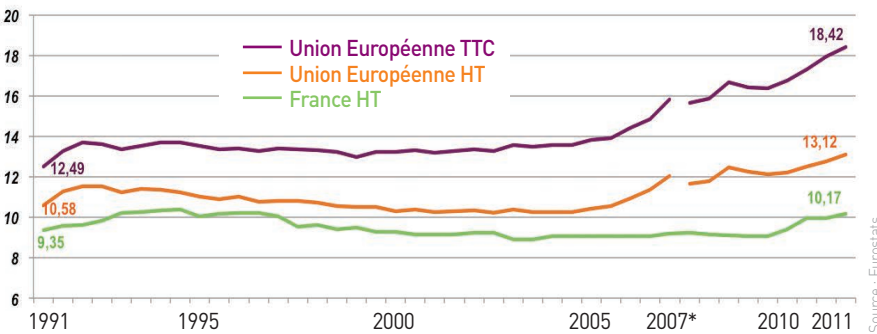
PRIX MOYEN DU KWH AUX CLIENTS DOMESTIQUES DE 1991 À 2011 (en cts d'€)
